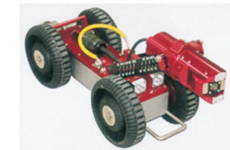
TVカメラロボット φ200mm~φ700mm
